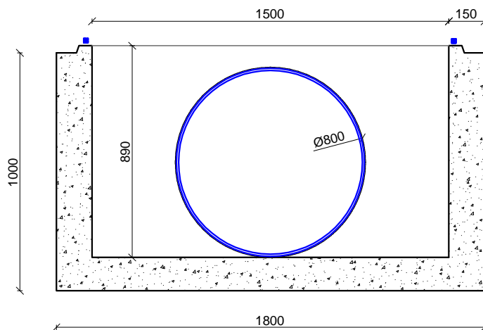
COUPE -AA-
