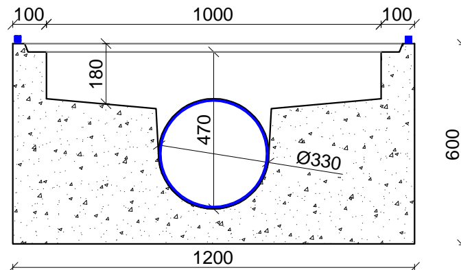
COUPE -AA-
